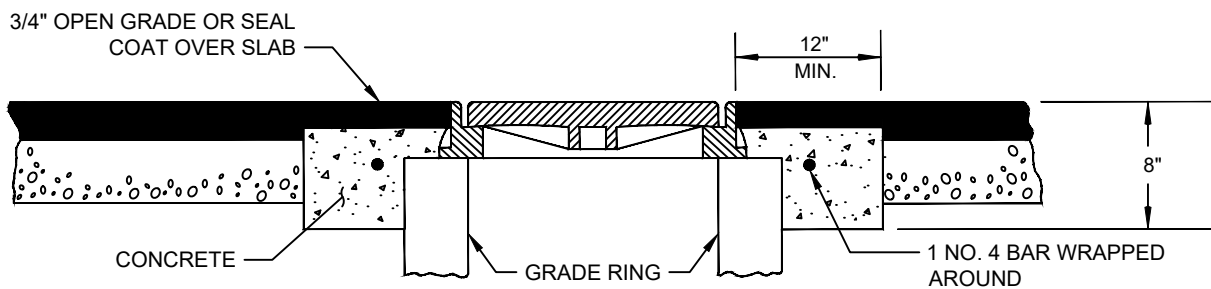
SECTION A-A
